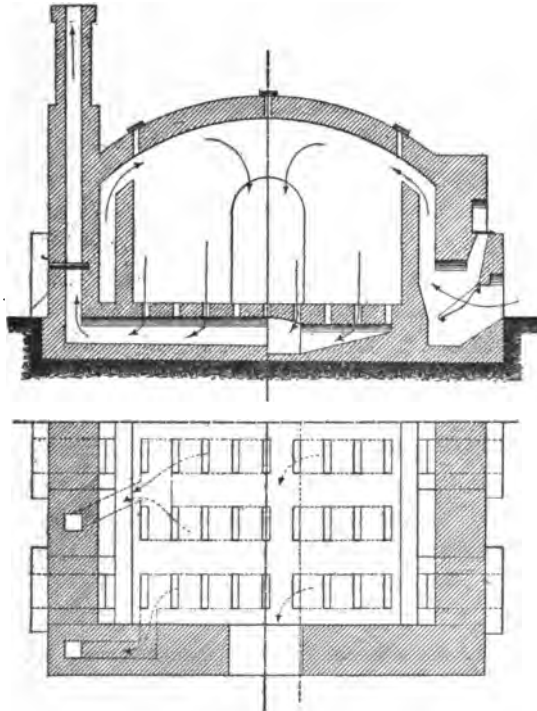
Fig. 174. — Four à flammes renversées.
